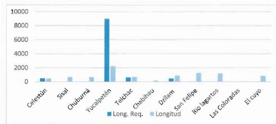
Figura 86 Longitud de Atraque vs Longitud de Atraque requerida para Flota Mayor
