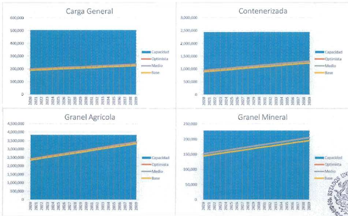
Figura 8 Comparativa de oferta y demanda por línea de negocio (2020-2039)
