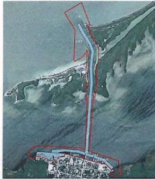
Figura 40 Obras de protección del Recinto de San Felipe
